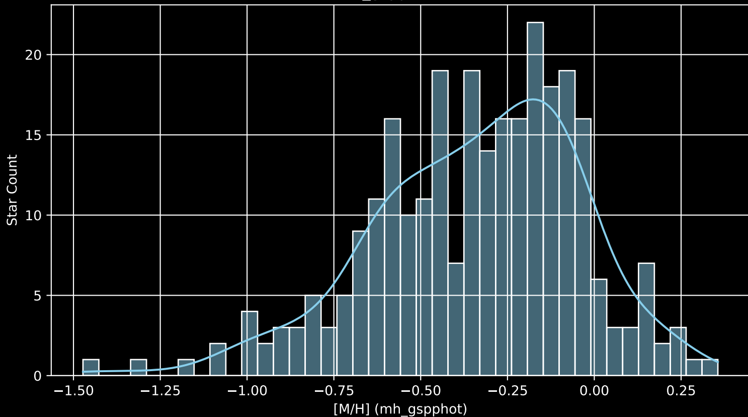
GALAH DR4 Field: [315] [M/H] (mh_gspphot) (n= 279)
