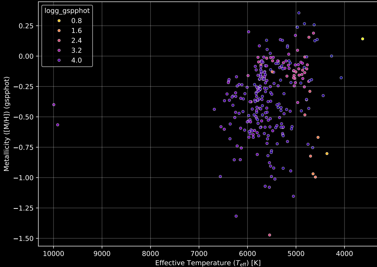
GALAH DR4 Field: [315] Stellar Population Parameters (n= 279)
