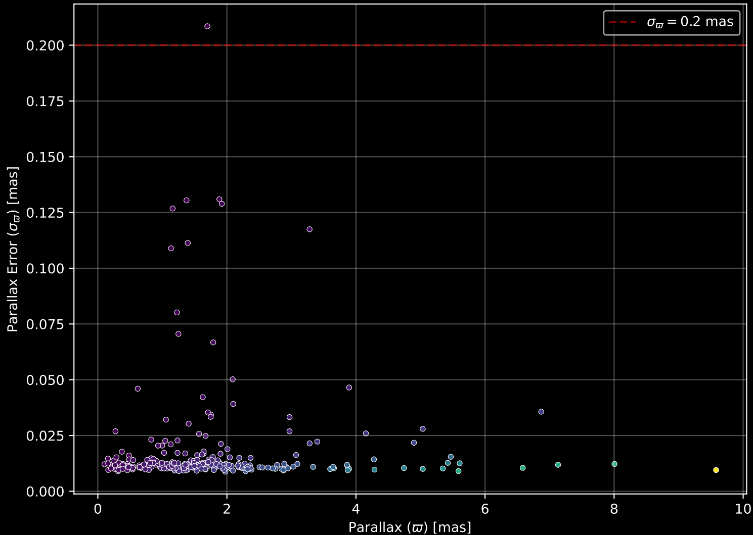
GALAH DR4 Field: [315] Parallax Quality (n= 279)
