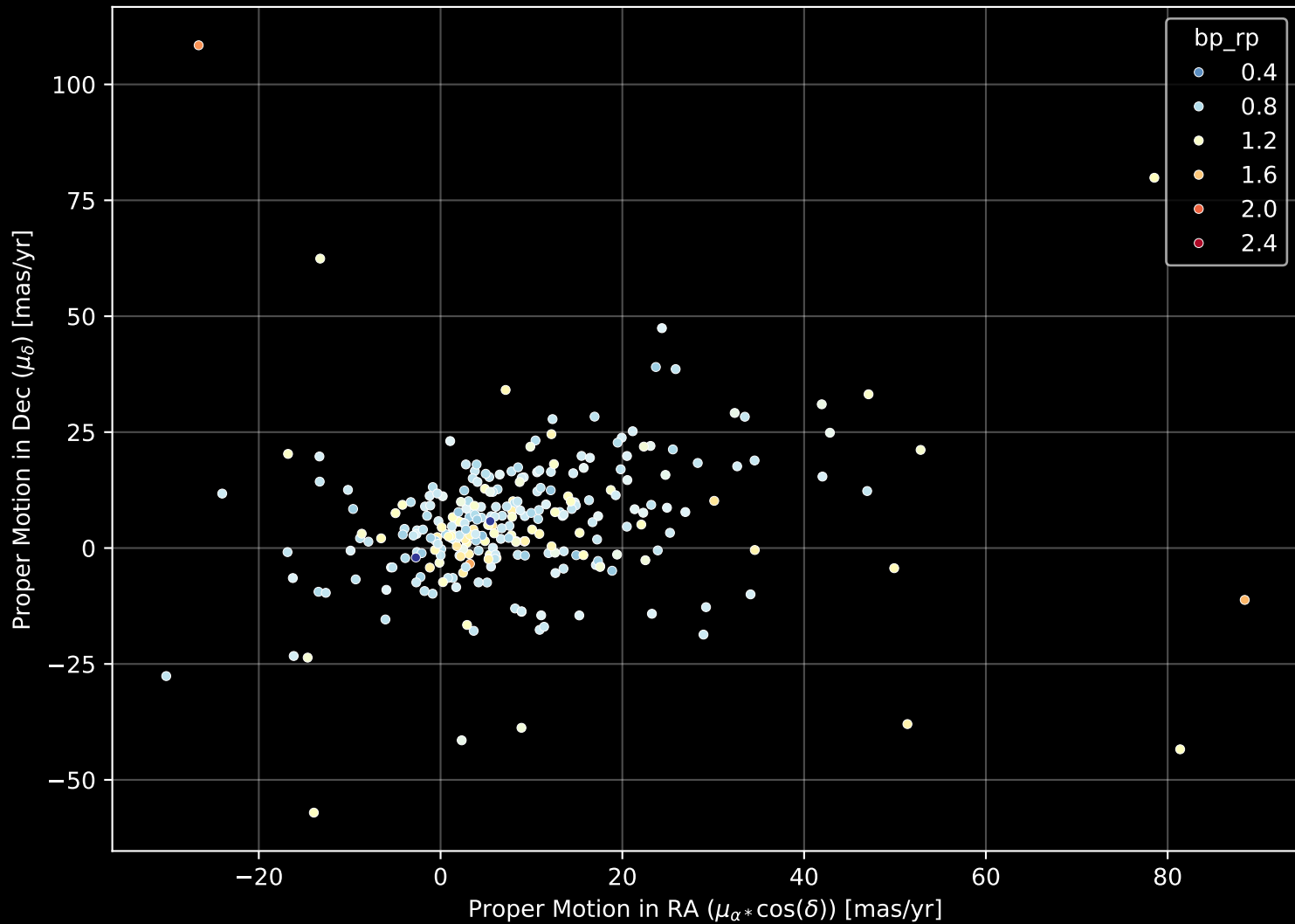
GALAH DR4 Field: [315] Proper Motion Diagram (n= 279)
