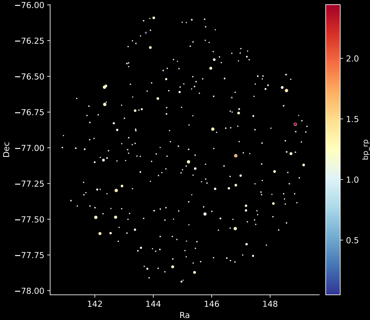
GALAH DR4 Field: [315] Stars: 279
